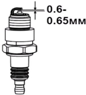
Рис. 15 Свеча зажигания
